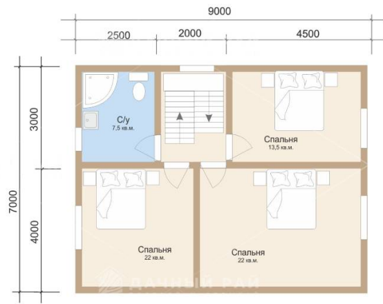
План 2 этажа
