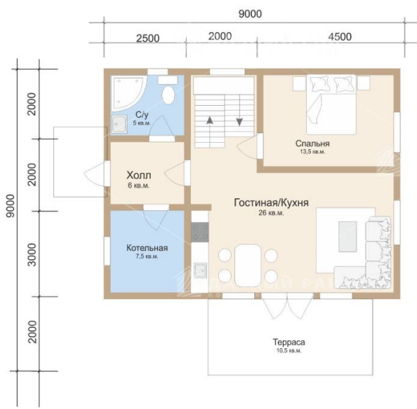
План 1 этажа
