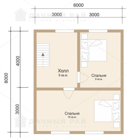
План 2 этажа
