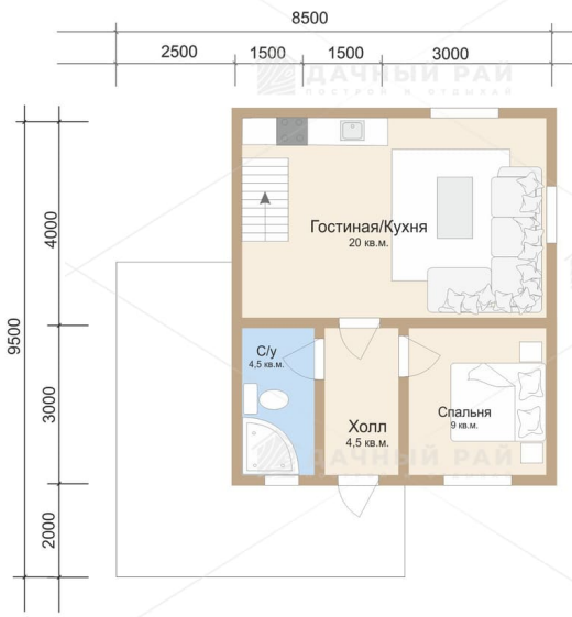
План 1 этажа
