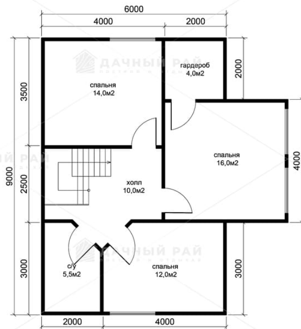
план 2-ого этажа
