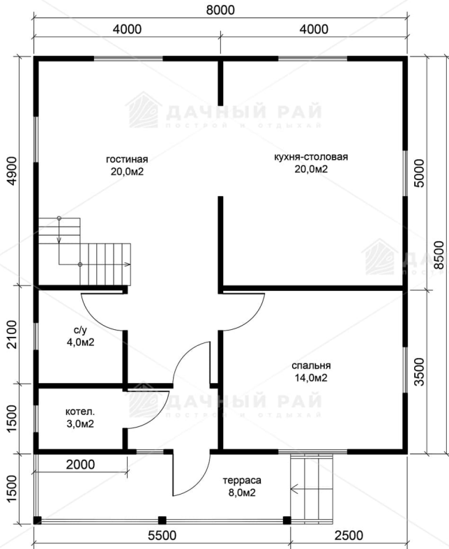
план 1-ого этажа
