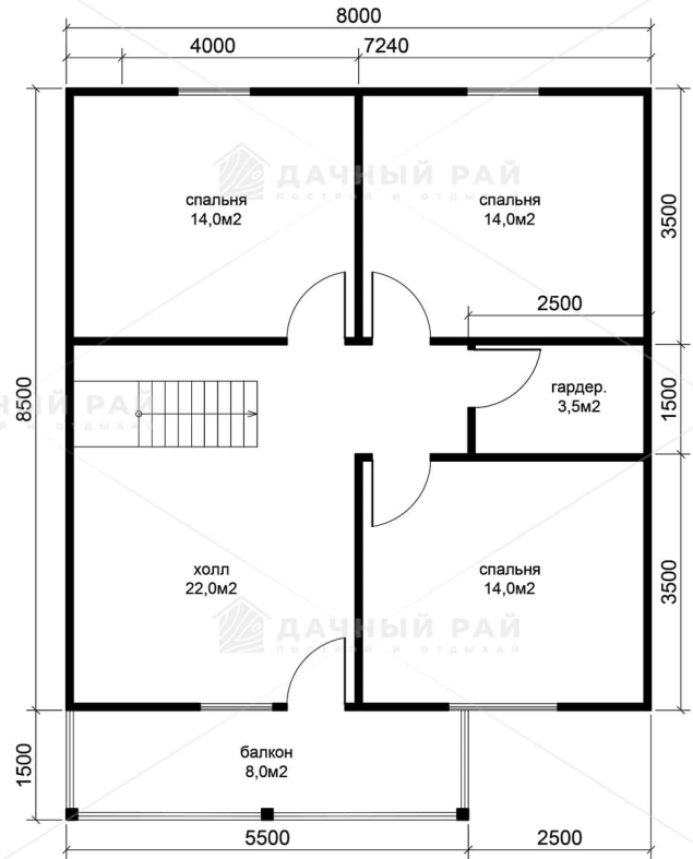
план 2-ого этажа
