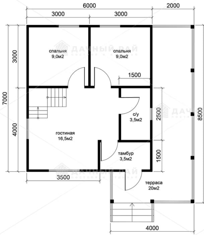
план 1-ого этажа
