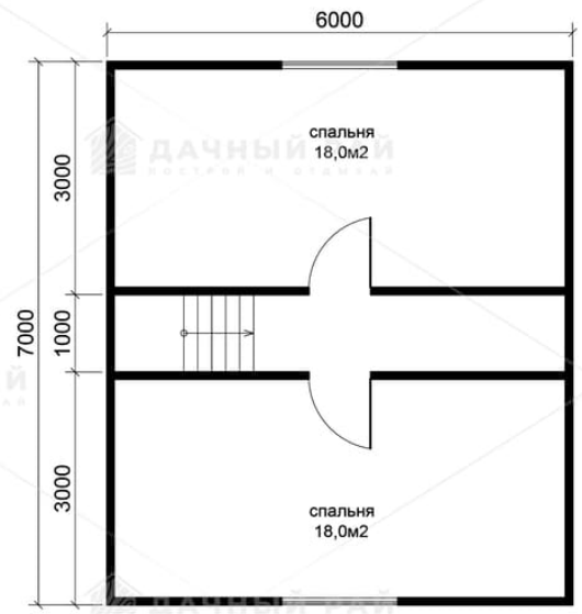
план 2-ого этажа
