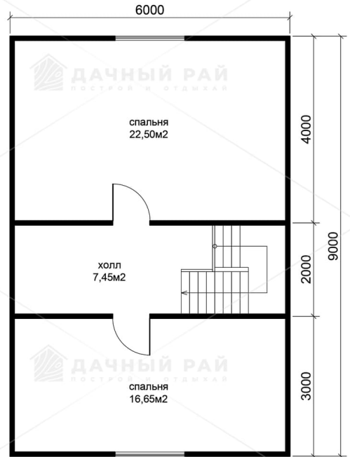
план 2-ого этажа
