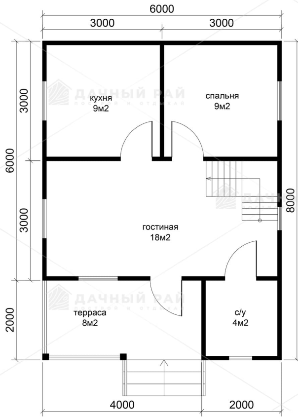
план 1-ого этажа
