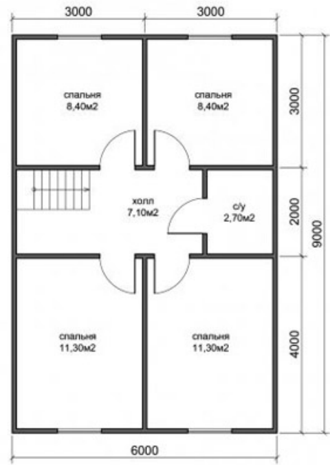
план 2-ого этажа
