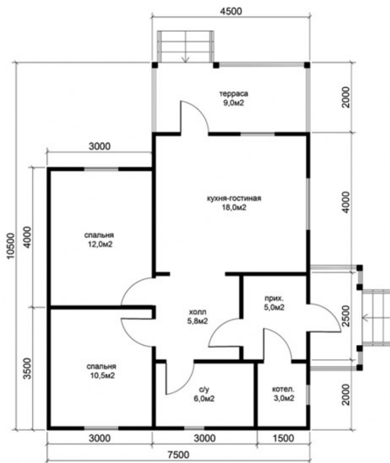
план 1-ого этажа
