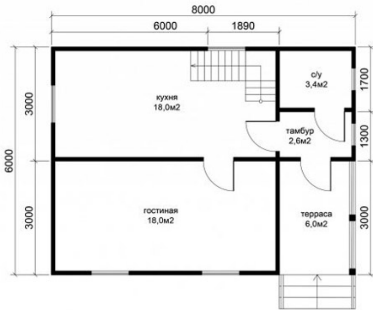
план 1-ого этажа
