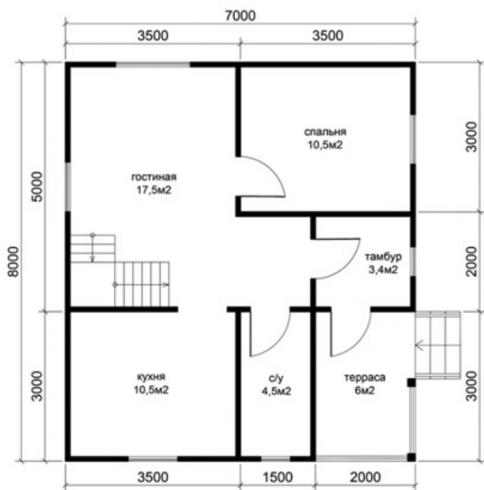
план 1-ого этажа
