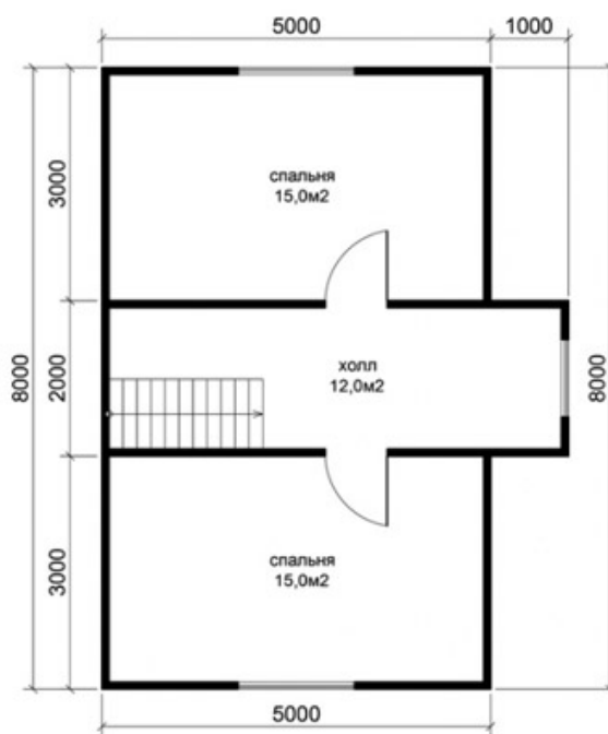
план 2-ого этажа
