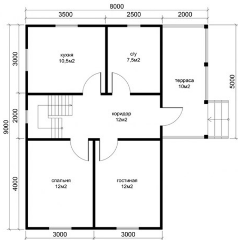
план 1-ого этажа
