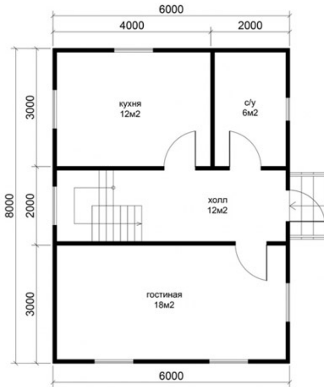
план 1-ого этажа
