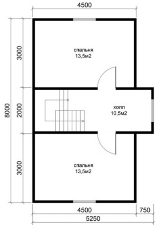
план 2-ого этажа
