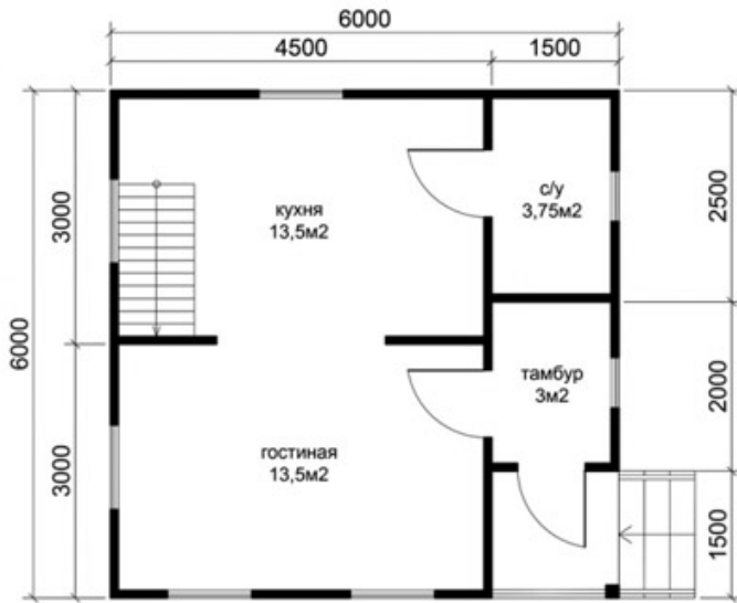
план 1-ого этажа
