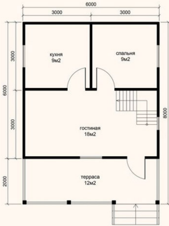
план 1-ого этажа
