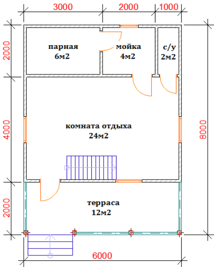
План 1-ого этажа
